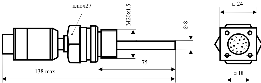
Рисунок 3. Термопреобразователь ТСП 001-03-75 модель 2 с 19 штырьковым разъемом
